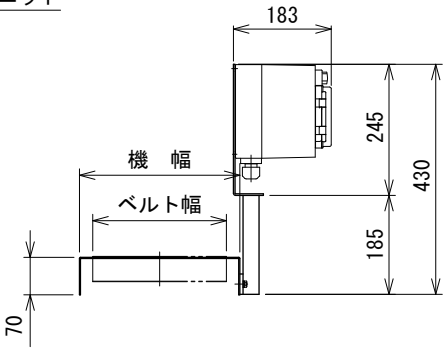
中間断面図
