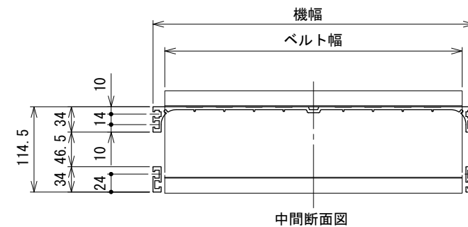
中間断面図
