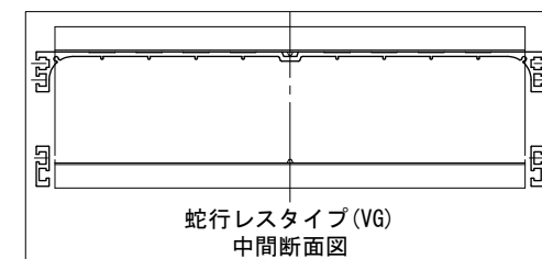
中間断面図
