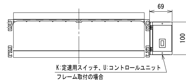
A-A矢視図
