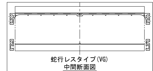
中間断面図
