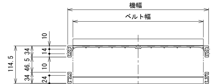
中間断面図
