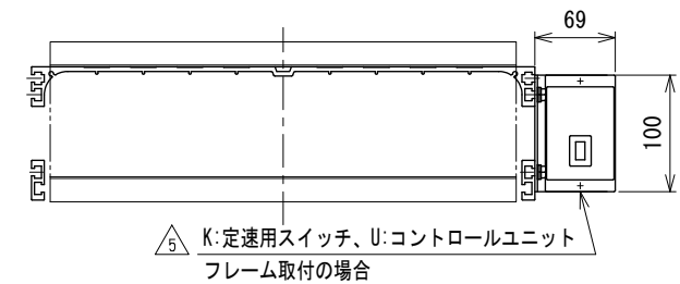
A-A矢視図
