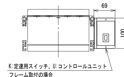
A-A矢視図
