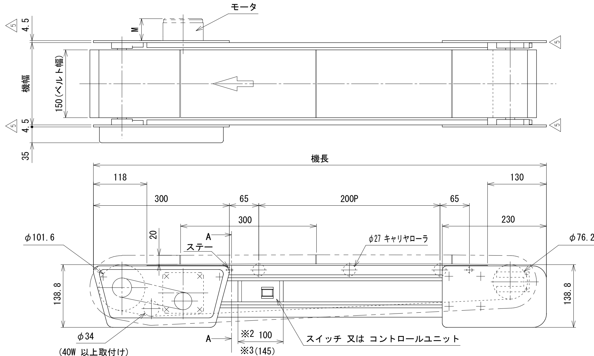
△5 モータ飛び出し寸法表 M(最大値) 単位 mm
