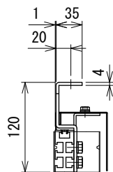
A-A 矢視図
