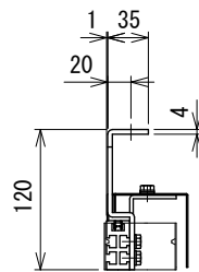
A-A 矢視図
