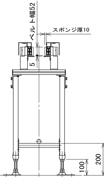
中間断面図
