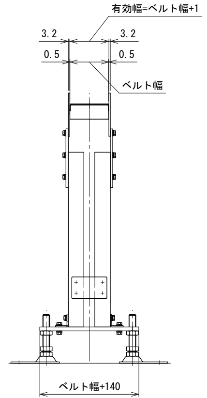
中間断面図
