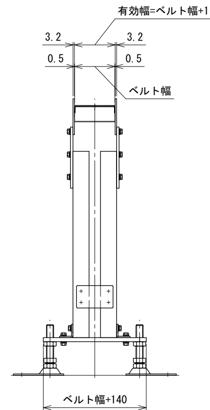
中間断面図
