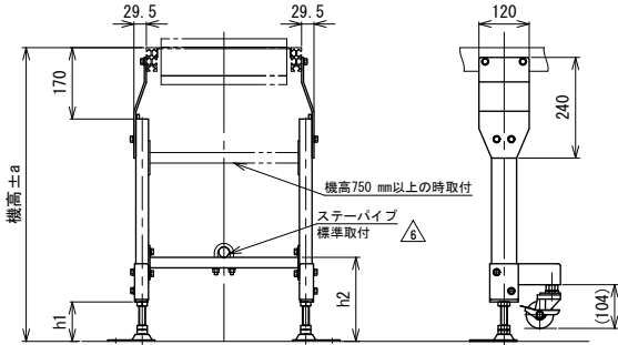
MB2S-HAC2 ベルト幅:300, 350, 400, 500, 600
