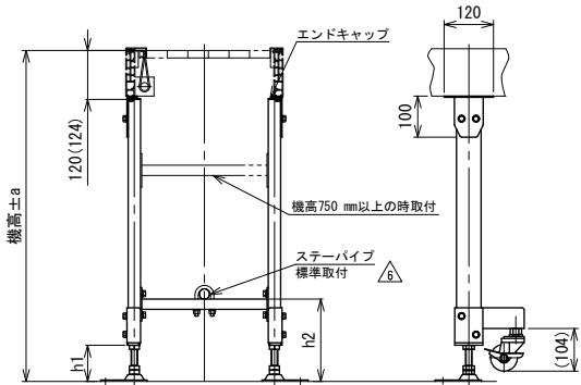
MRA2-HAC2 ローラ幅:700, 800
