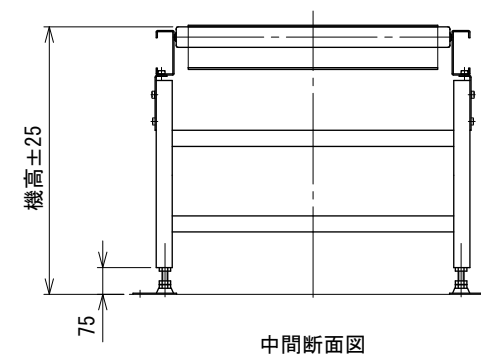
中間断面図
