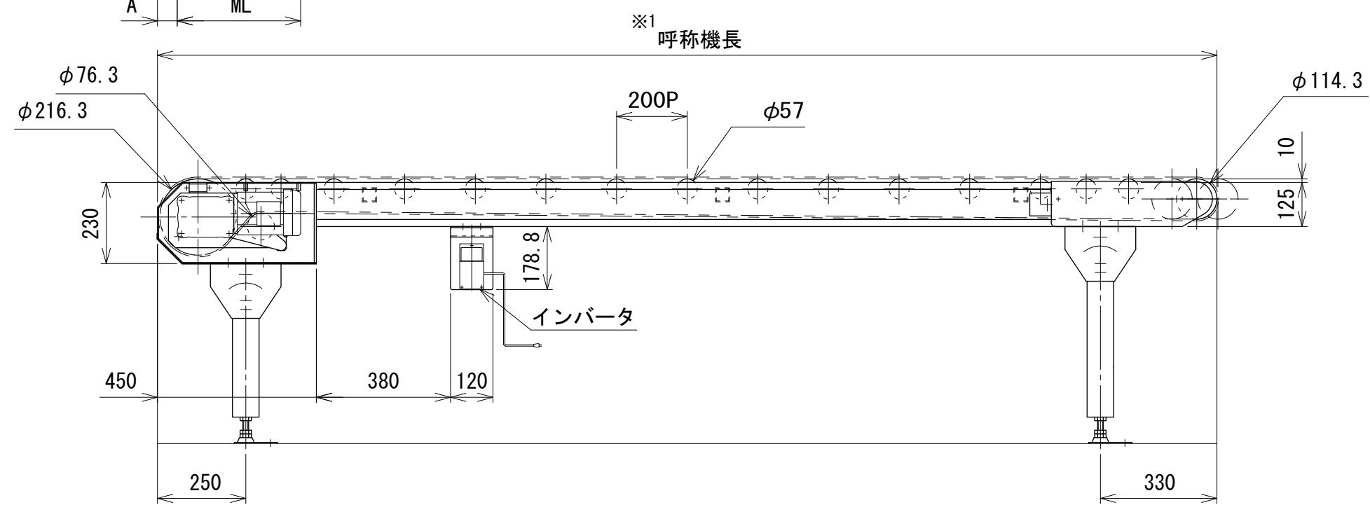
モータ関連寸法表 単位 mm
