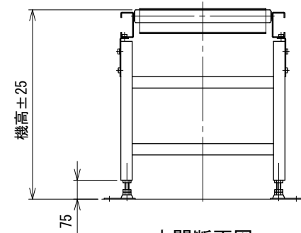
中間断面図
