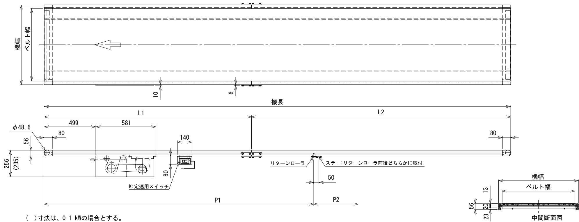
フレーム分割, リターンローラ取付寸法表
