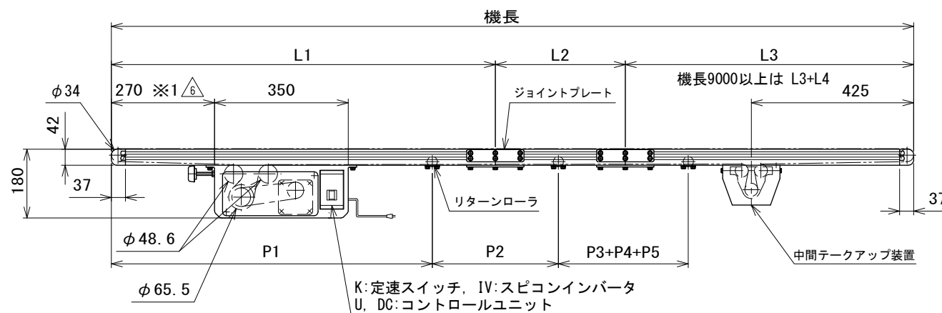
フレーム分割, リターンローラ取付寸法表 △6
