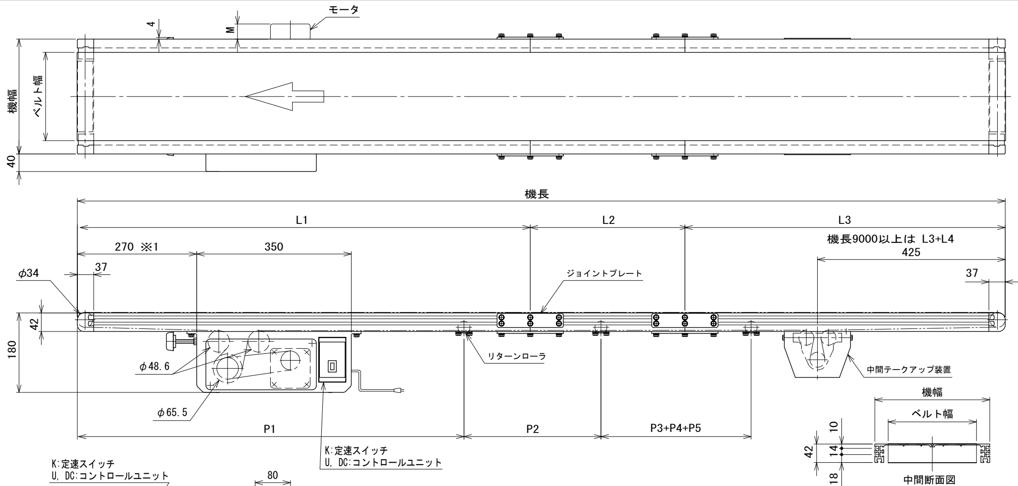
フレーム分割、リターンローラ取付寸法表
