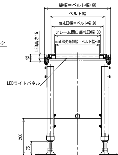
中間断面図
