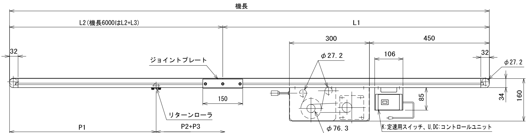
フレーム分割, リターンローラ取付寸法表
