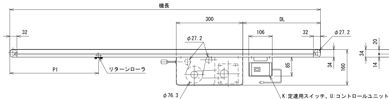
原動位置寸法表
