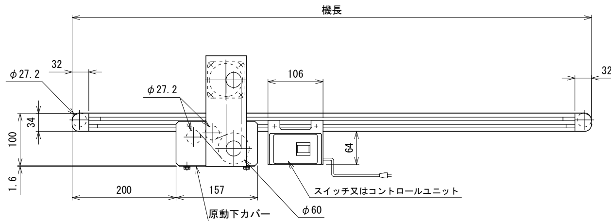
原動部寸法表 単位 mm
