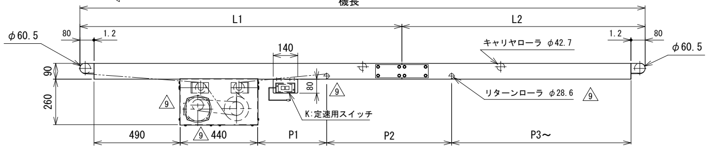
フレーム分割, リターンローラ取付寸法表
