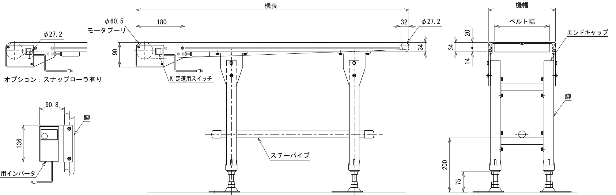
中間断面図
