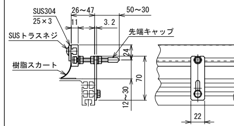
SG6-A 材質:ガイド…樹脂スカート, ブラケット…鉄(メッキ) ガイド幅調節式
