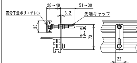
SG6 材質:ガイド…樹脂スカート, ブラケット…鉄(メッキ) ガイド幅固定式
