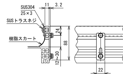
SG6-A 材質:ガイド…樹脂スカート, ブラケット…鉄(メッキ) ガイド幅調節式
