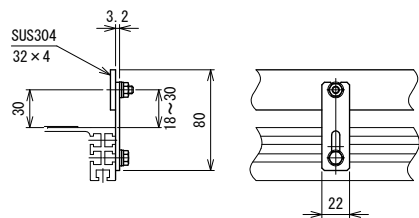
SG1 材質:ガイド…ステンレス, ブラケット…鉄(メッキ) ガイド幅固定式
