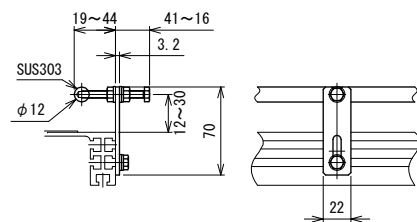
SG3 材質:ガイド…樹脂, ブラケット…鉄(メッキ) ガイド幅固定式
