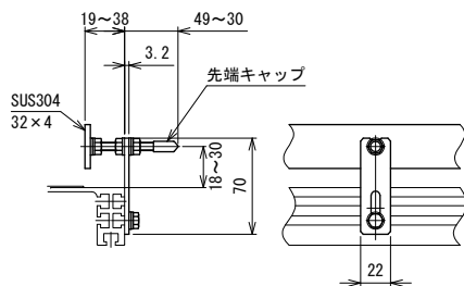
SG2 材質:ガイド…ステンレス, ブラケット…鉄(メッキ) ガイド幅固定式
