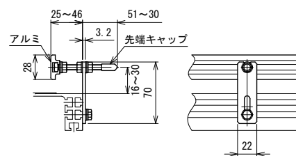
SG5 材質:ガイド…樹脂, ブラケット…鉄(メッキ) ガイド幅固定式
