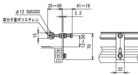
SG3-A 材質:ガイド…樹脂, ブラケット…鉄(メッキ) ガイド幅調節式
