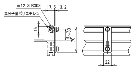
SG3-A 材質:ガイド…樹脂, ブラケット…鉄(メッキ) ガイド幅調節式
