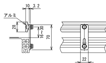
SG4-A 材質:ガイド…アルミ, ブラケット…鉄(メッキ) ガイド幅調節式
