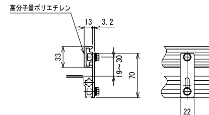
SG5 材質:ガイド…樹脂, ブラケット…鉄(メッキ) ガイド幅固定式
