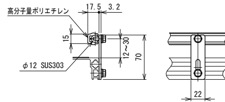
SG3-A 材質:ガイド…樹脂, ブラケット…鉄(メッキ) ガイド幅調節式
