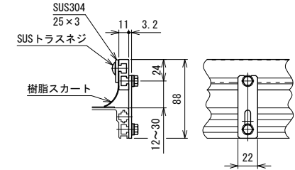
SG6-A 材質:ガイド…樹脂スカート, ブラケット…鉄(メッキ) ガイド幅調節式
