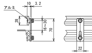
SG4 材質:ガイド…アルミ, ブラケット…鉄(メッキ) ガイド幅固定式
