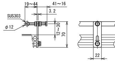
SG2-A 材質:ガイド…ステンレス, ブラケット…鉄(メッキ) ガイド幅調節式
