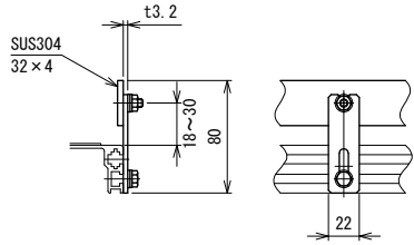
SG1 材質:ガイド…ステンレス, ブラケット…鉄(メッキ) ガイド幅固定式
