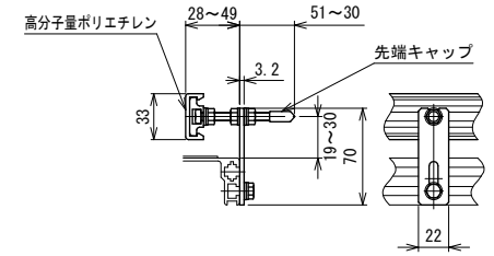
SG5-A 材質:ガイド…樹脂, ブラケット…鉄(メッキ) ガイド幅調節式
