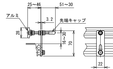
SG5 材質:ガイド…樹脂, ブラケット…鉄(メッキ) ガイド幅固定式
