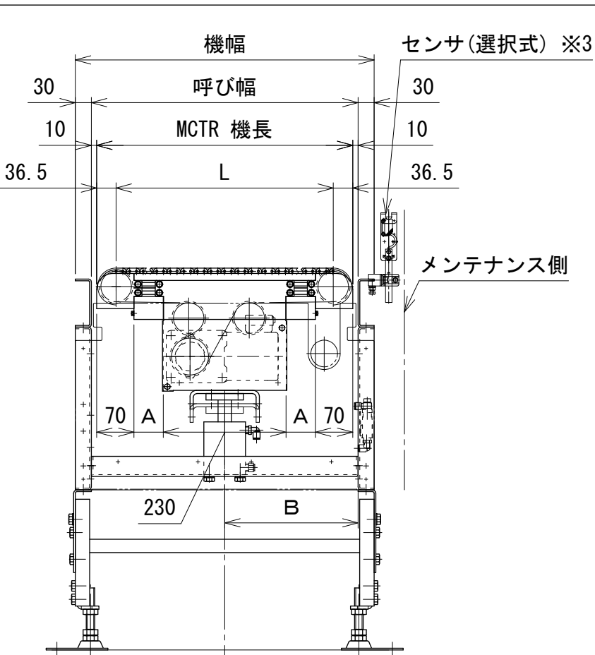
A-A矢視図
