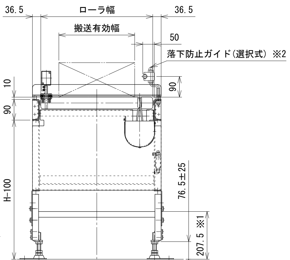
A-A矢視図
