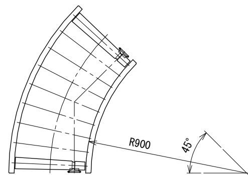
相当ローラピッチ100
