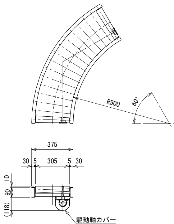
相当ローラピッチ75
