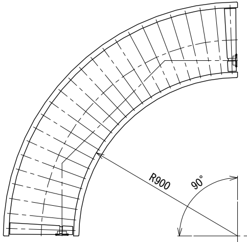
相当ローラピッチ75
