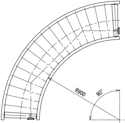
相当ローラピッチ100
