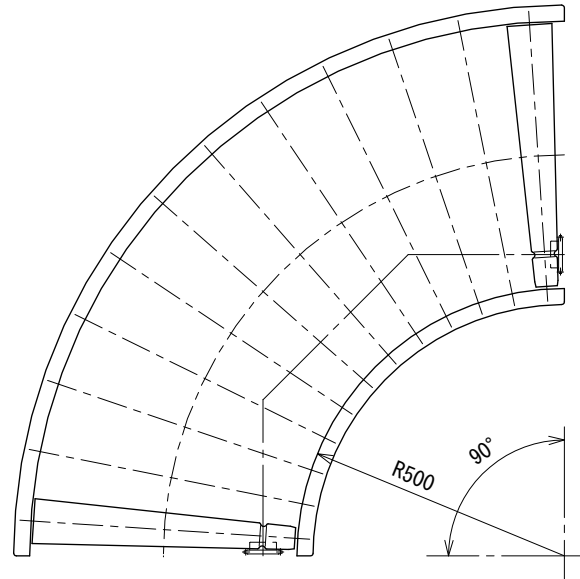
相当ローラピッチ75
