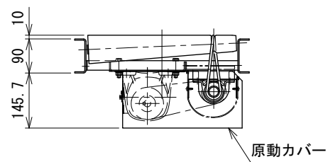
原動部断面図
