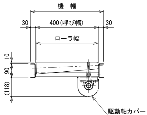
中間断面図
