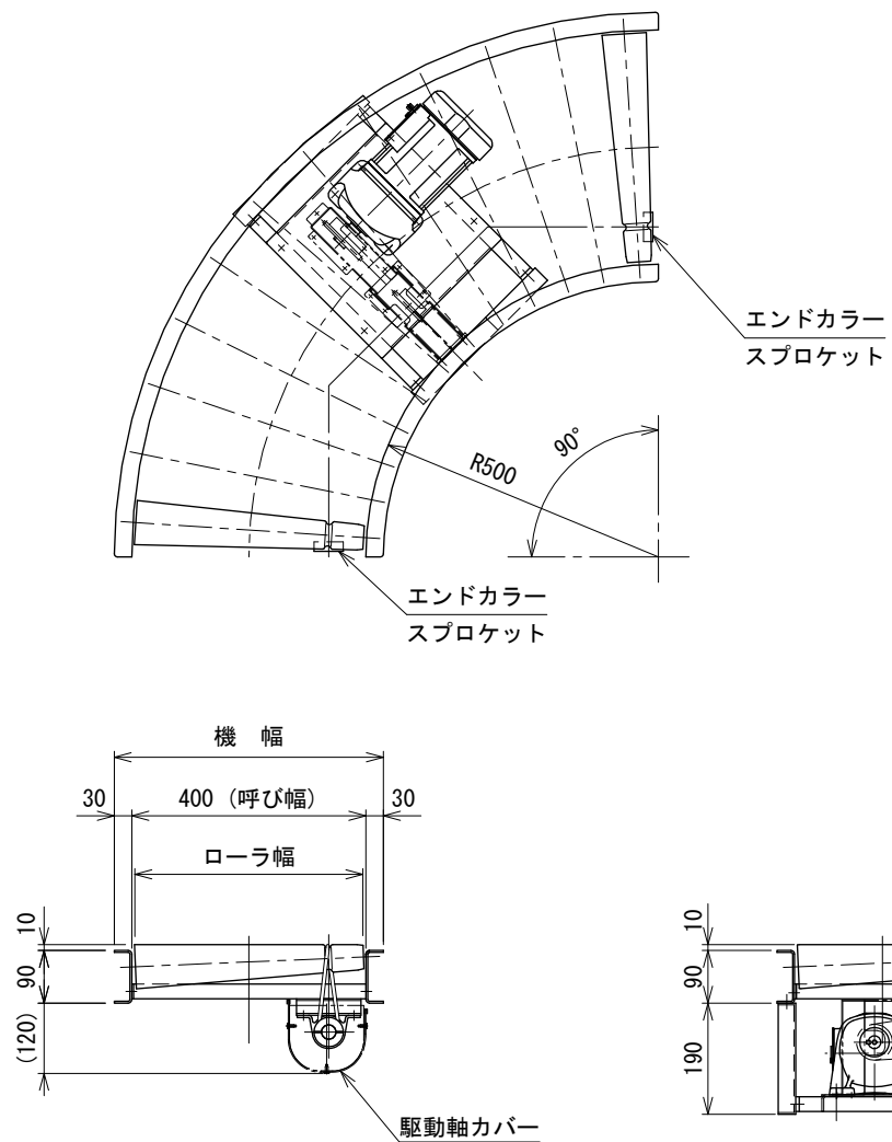
原動部断面図
