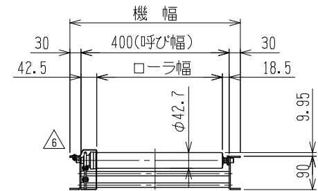
中間断面図
