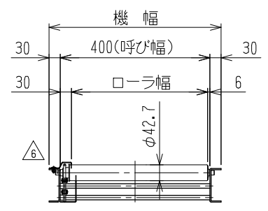
中間断面図
