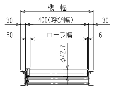
中間断面図
