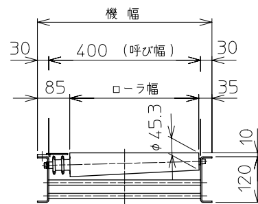
一般断面図
