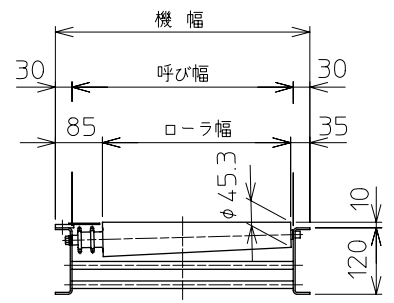
一般断面図
