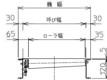
一般断面図
