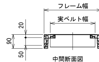
中間断面図
