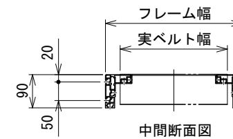
中間断面図
