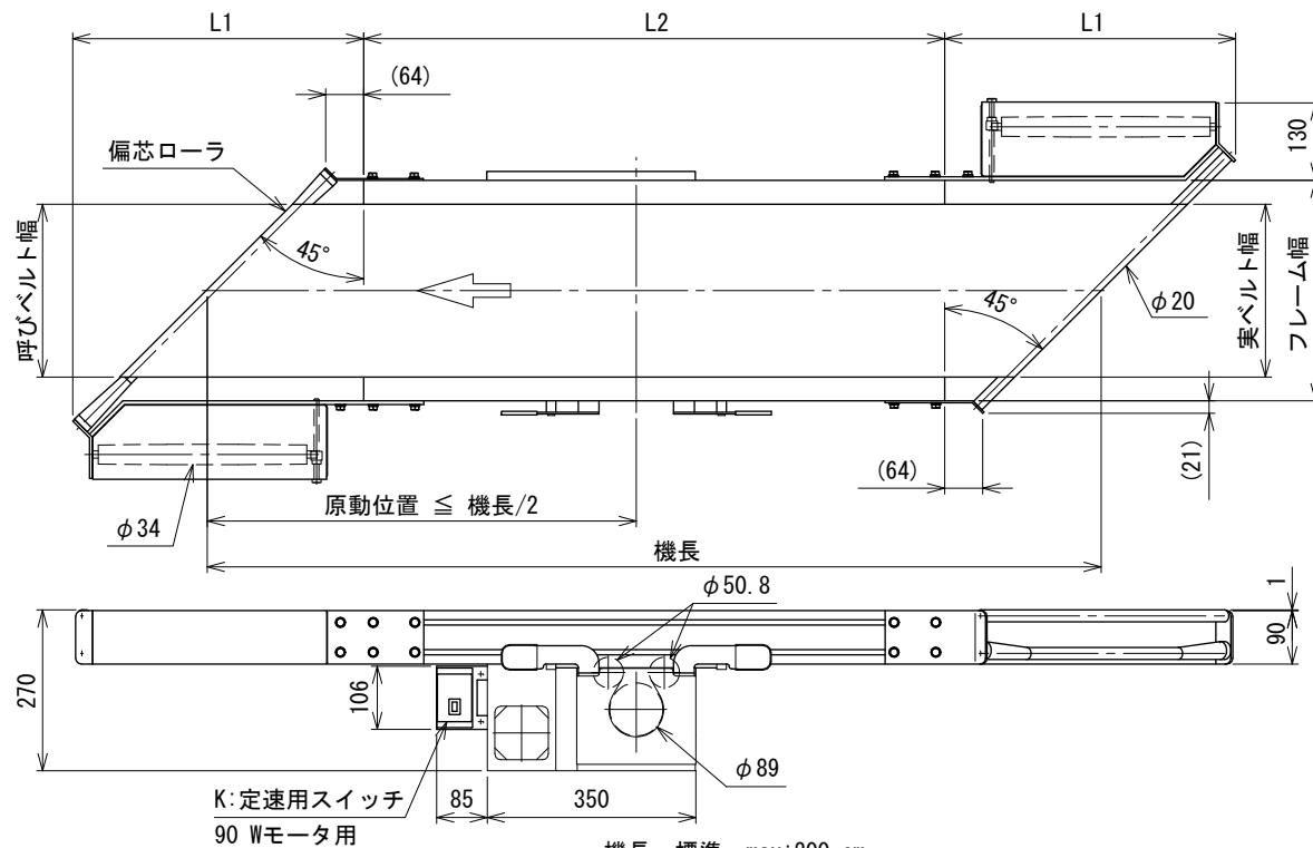
テール部角度 45° タイプ (菱形タイプ)
