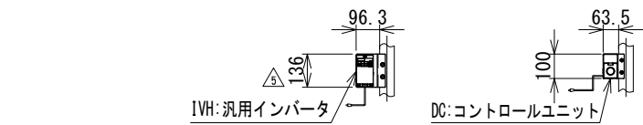
モータ関連寸法表 単位 mm
