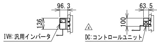
モータ関連寸法表 単位 mm
