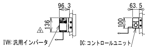
モータ関連寸法表 単位 mm
