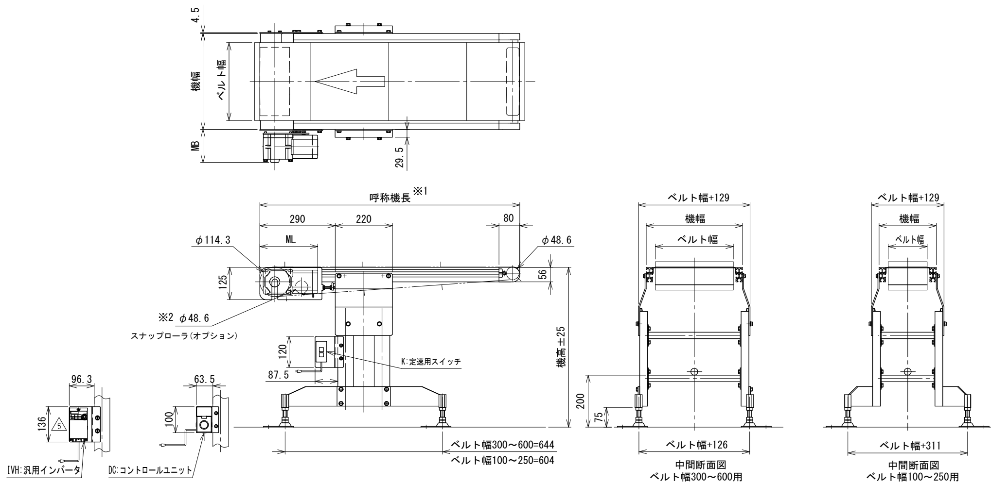
モータ関連寸法表 単位 mm
