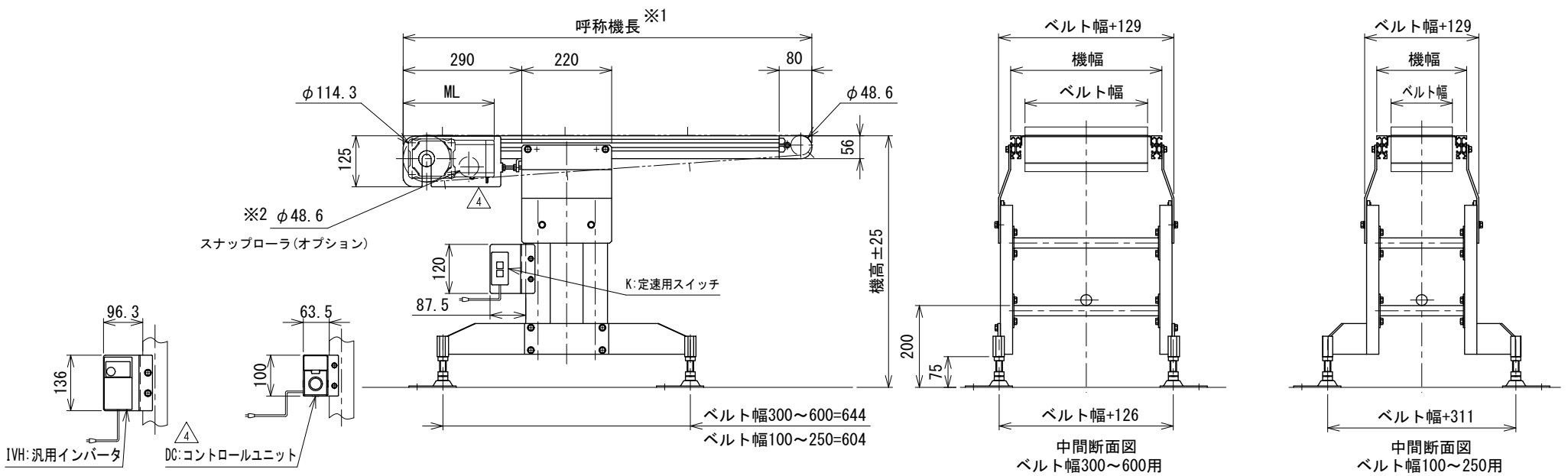
モータ関連寸法表 単位 mm
