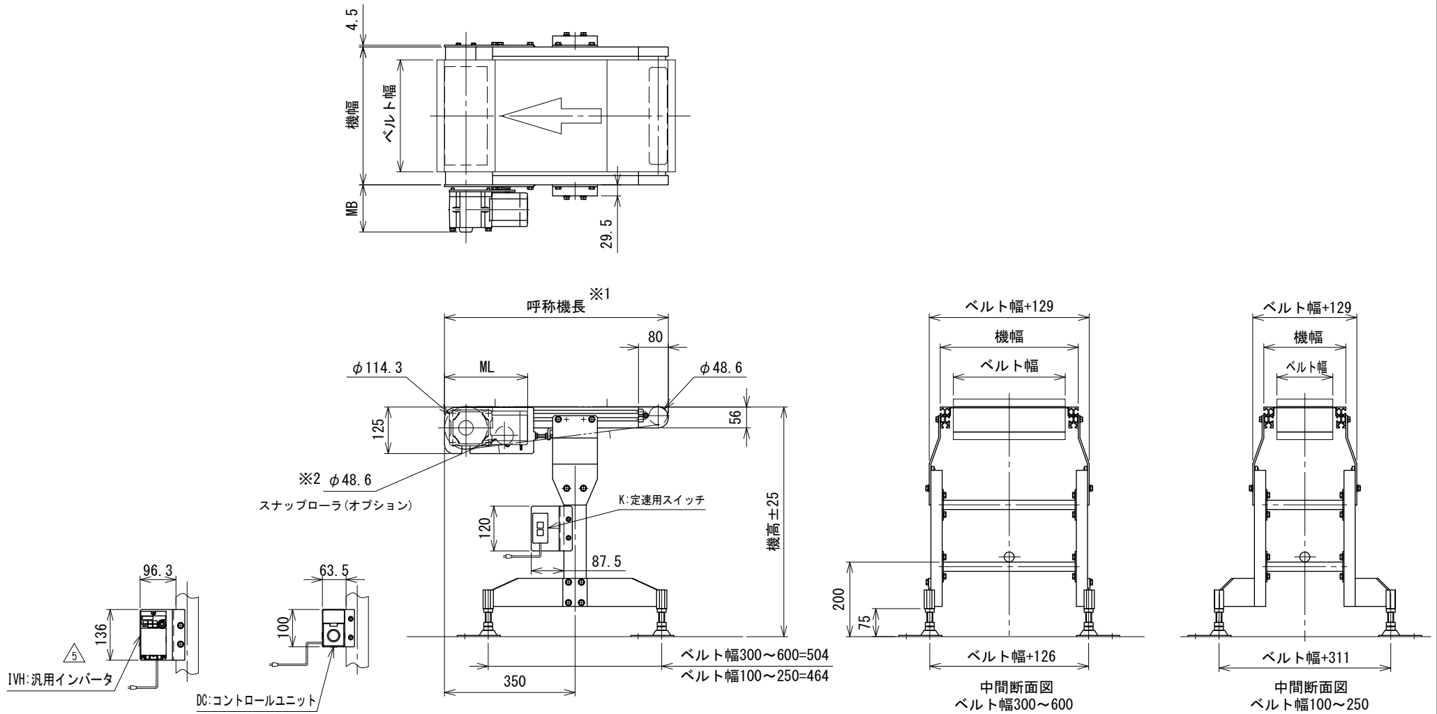
モータ関連寸法表 単位 mm
