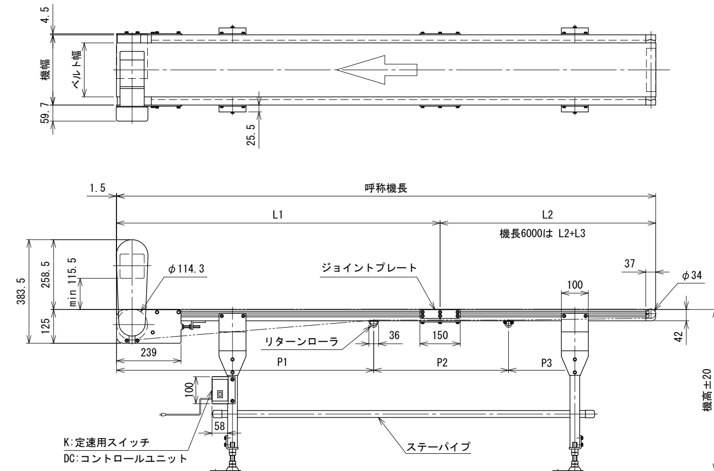
フレーム分割, リターンローラ取付寸法表
