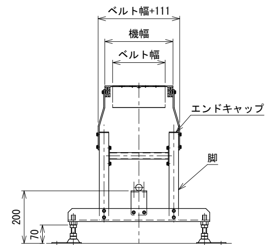
中間断面図
