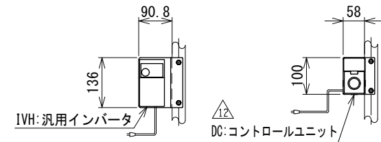
モータ関連寸法表 単位 mm
