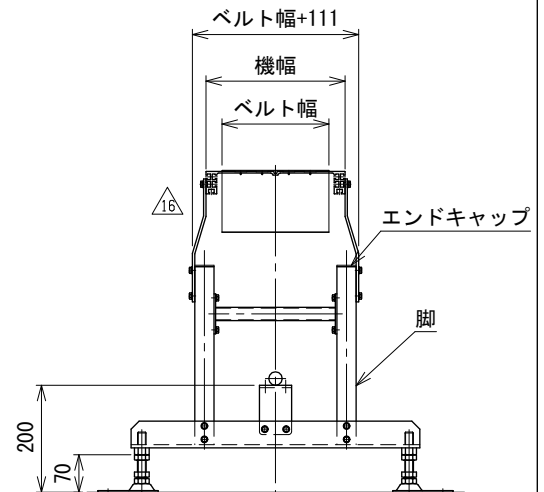
中間断面図
